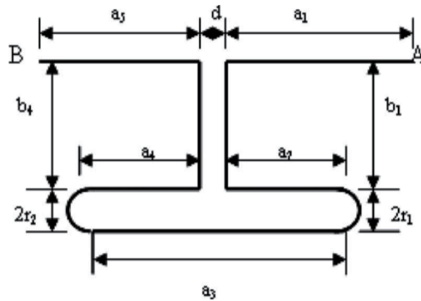
Fig. 31. T-spring Dimensions
